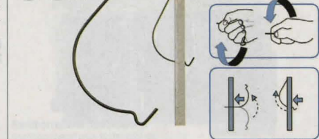
Gipskrok Hercules För montage i gipsskiva, inga verktyg krävs. Monteras med handkraft och lämnar endast ett litet hål. Total längd 105 mm, utstickande del 15 mm. 5-pack. 31-4620 ..... 39:-
