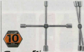
Fällbart fälgkors Cocraft Av kromvanadiumstål. Fällbart fälgkors med låsknapp. För hjulmuttrar 17, 19, 21 och 23 mm.
