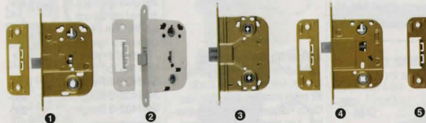
Låshus innerdörrar Alla utom 31-3424 har nyckelhål under. Vändbart tryckesfall för höger- och vänsterhängda innerdörrar. Kan förses med enbart dörrhandtag men även med toalett-/nyckelskylt. 31-3424 lev. utan slutbleck.
