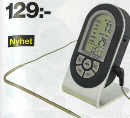
Stektermometer Underlätta matlagningen med en digital termometer. Inställbar och mäter temperatur upp till +300°C. Drivs med 2 x AAA/LR03-batterier (säljs separat). 44-1075 ..... 129:-
