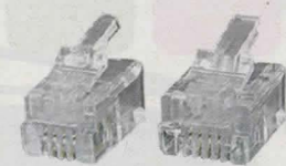
Modularkontakt För telefoner, telefonsvarare m.m. Levereras i 10-pack. Nr 1 förp. 10 förp. 22-4121 4P4C 7,5 mm..... 15:- 130:- 22-4122 6P4C 9,5 mm ..... 15:- 130:-
