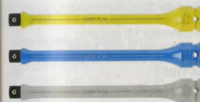
Momentstavar 1/2" för åtdragning med knackande mutterdragare till förutbestämt moment vid hjulbyte.
