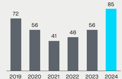
Utsläpp av växthusgaser, scope 1, ton CO 2 e
